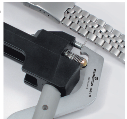
Retirer Herausziehen Remove Quitar
