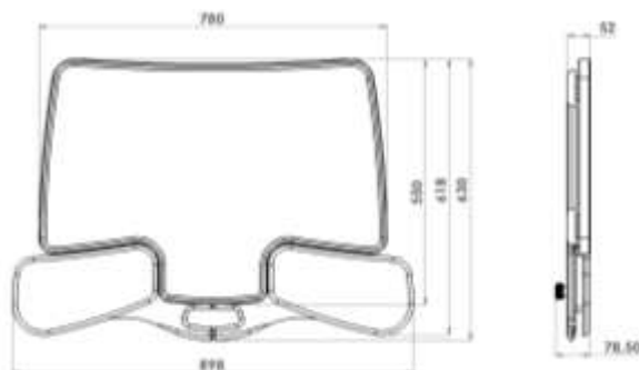
Etabli plié
